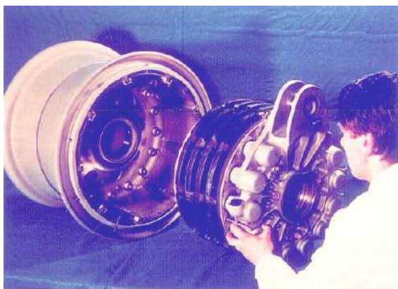
Discos de freio: atrito eleva a temperatura a 260 graus
